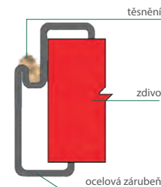
PROFIL OCELOVÉ ZÁRUBNĚ PRO DPB2
